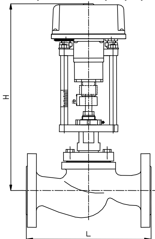
Рисунок 1. Габаритные установочные и присоединительные размеры клапана.
