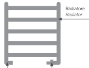
Detentore sinistro Left lockshield Valvola termostatica o manuale destra Thermostatic valve or right manual
