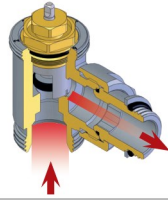
Valvola termostatica o manuale sinistra Thermostatic valve or left manual Detentore destro Right lockshield
