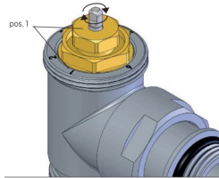
Detentore sinistro Left lockshield Valvola termostatica o manuale destra Thermostatic valve or right manual
