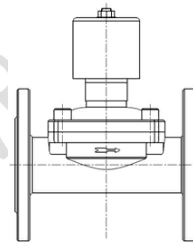
Рисунок 1. Устройство
